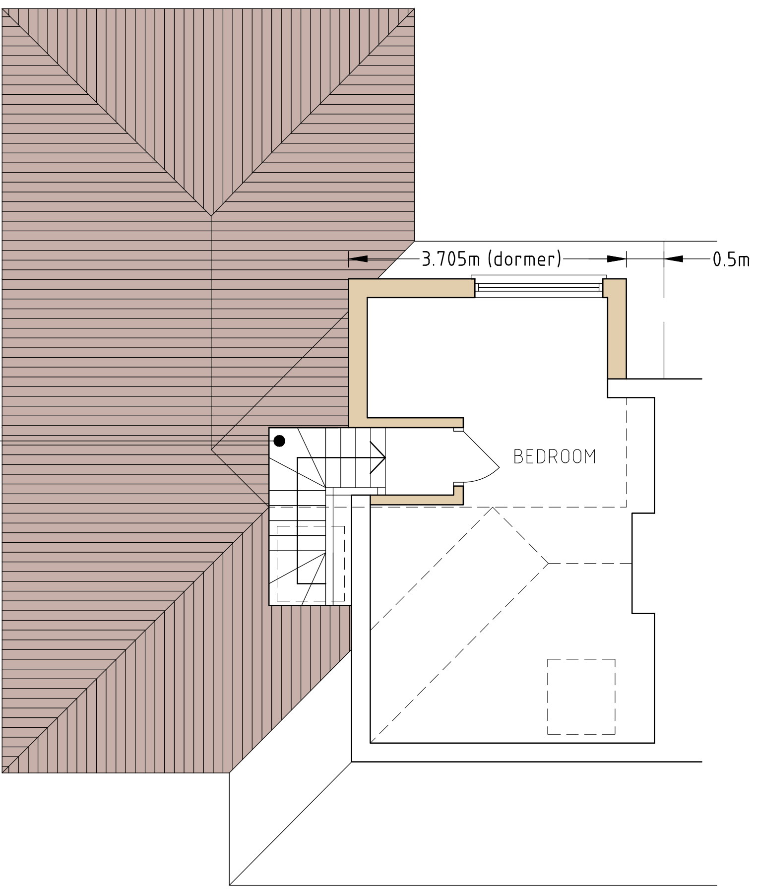
LOFT PLAN
