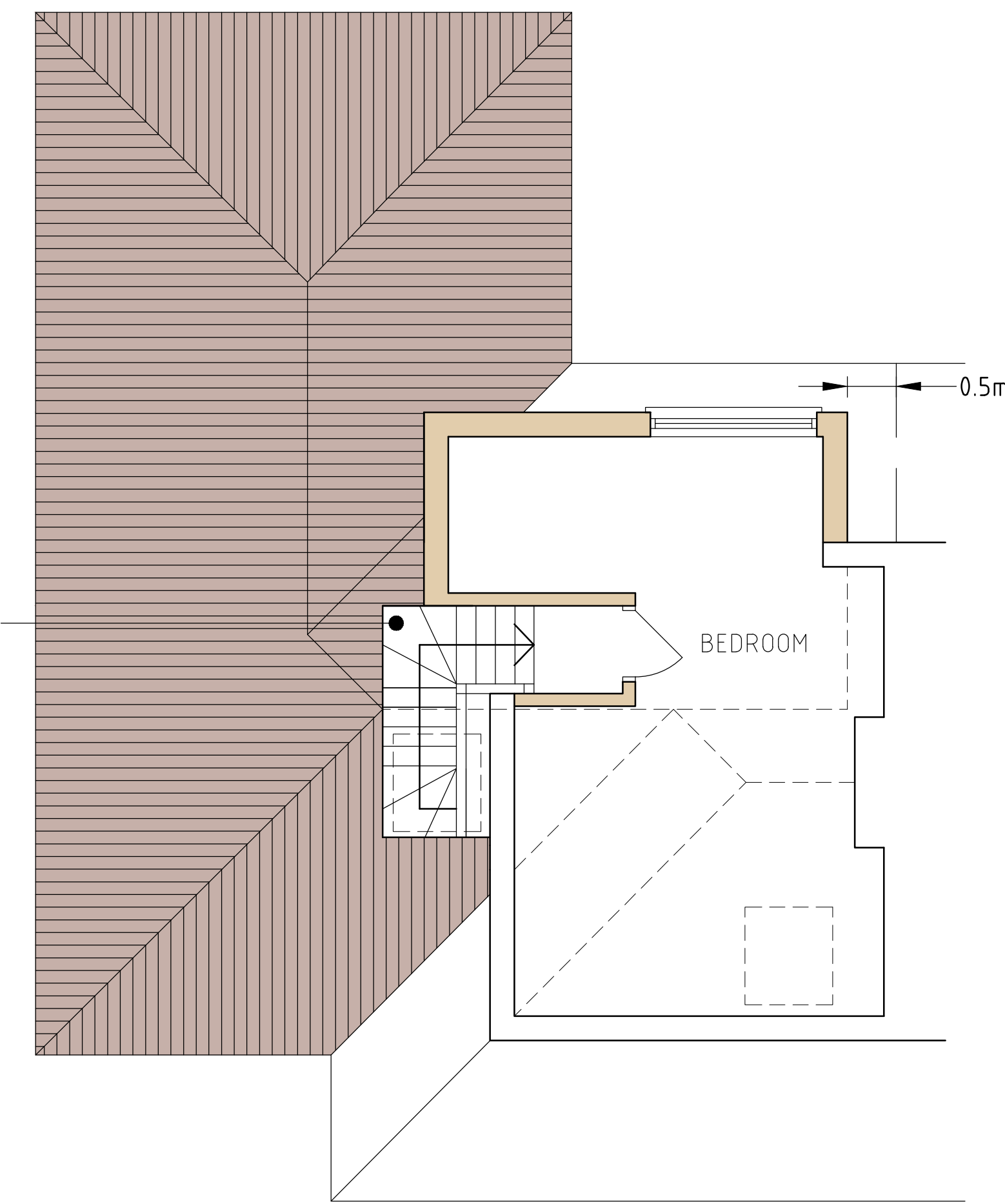
LOFT PLAN
