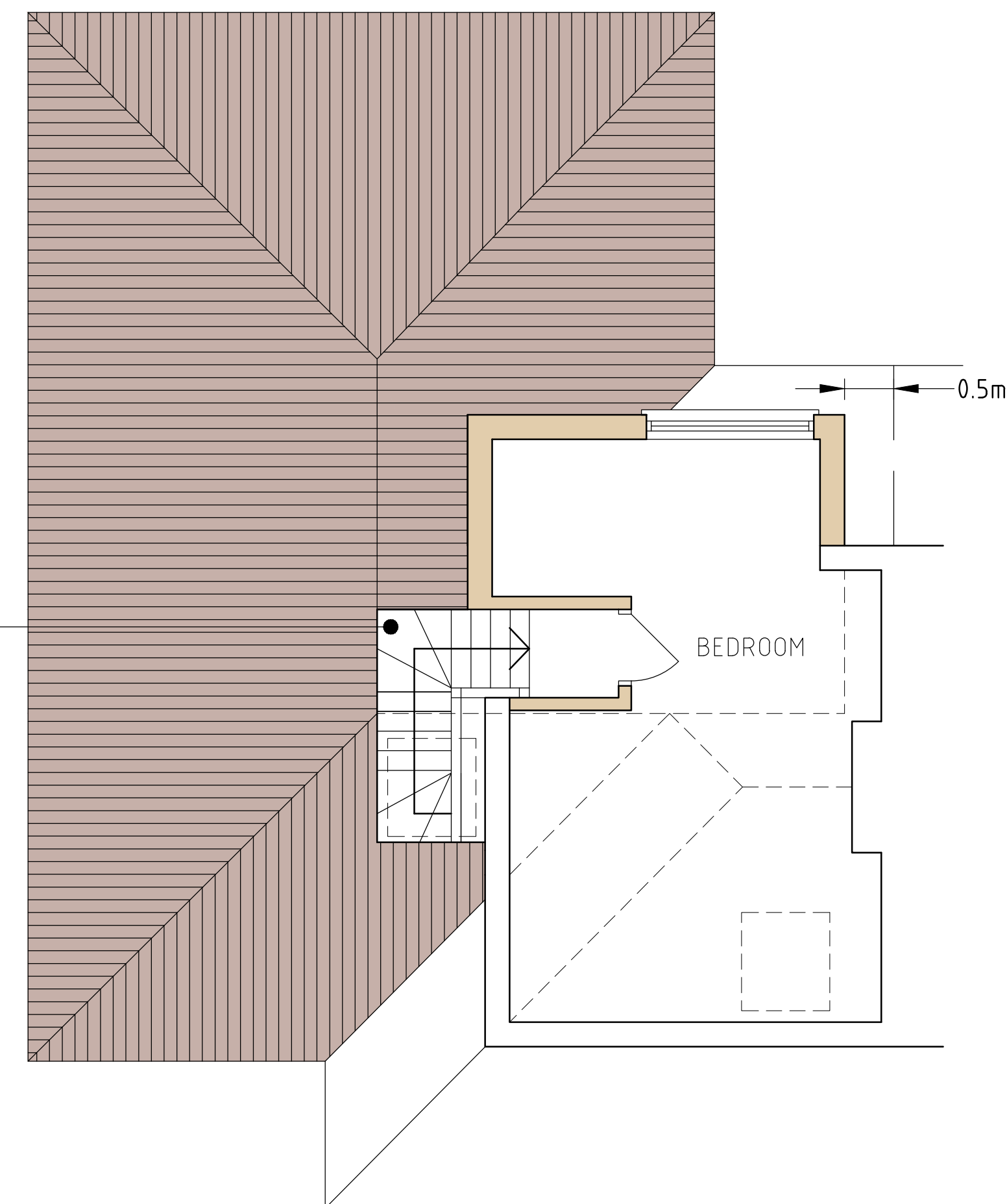
LOFT PLAN
