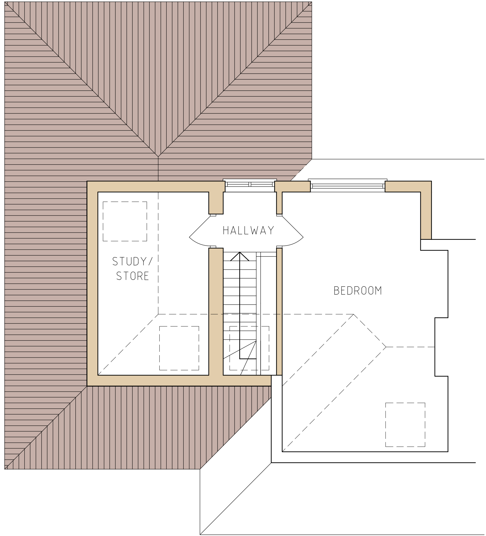
LOFT PLAN
