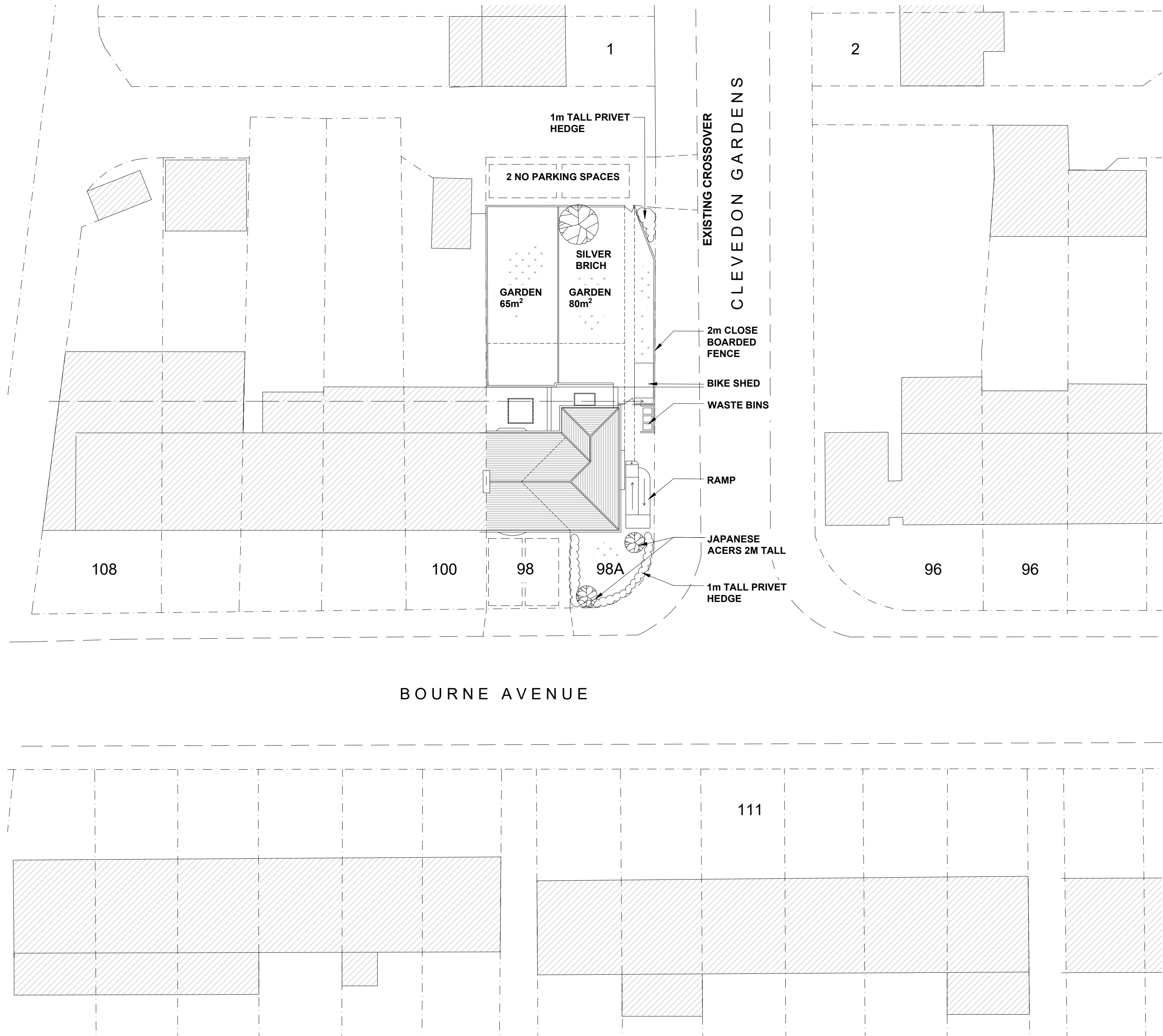
SITE PLAN 1:200
