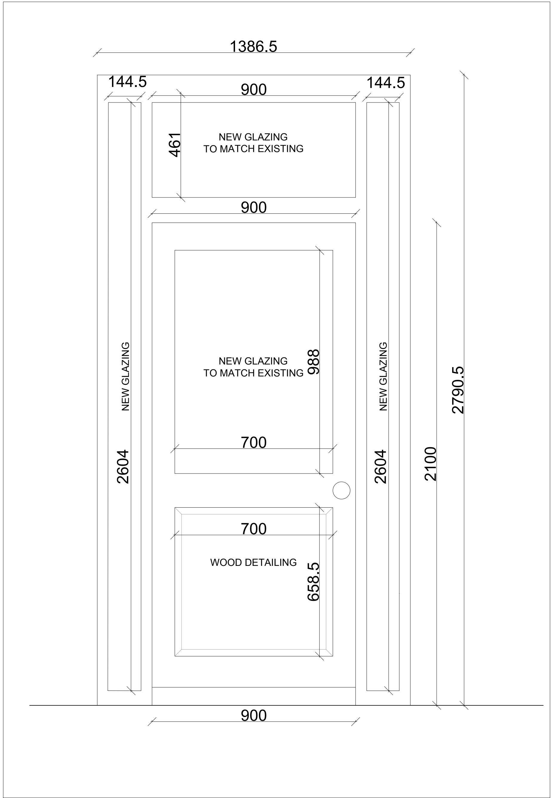
1:10 DOOR ELEVATION
