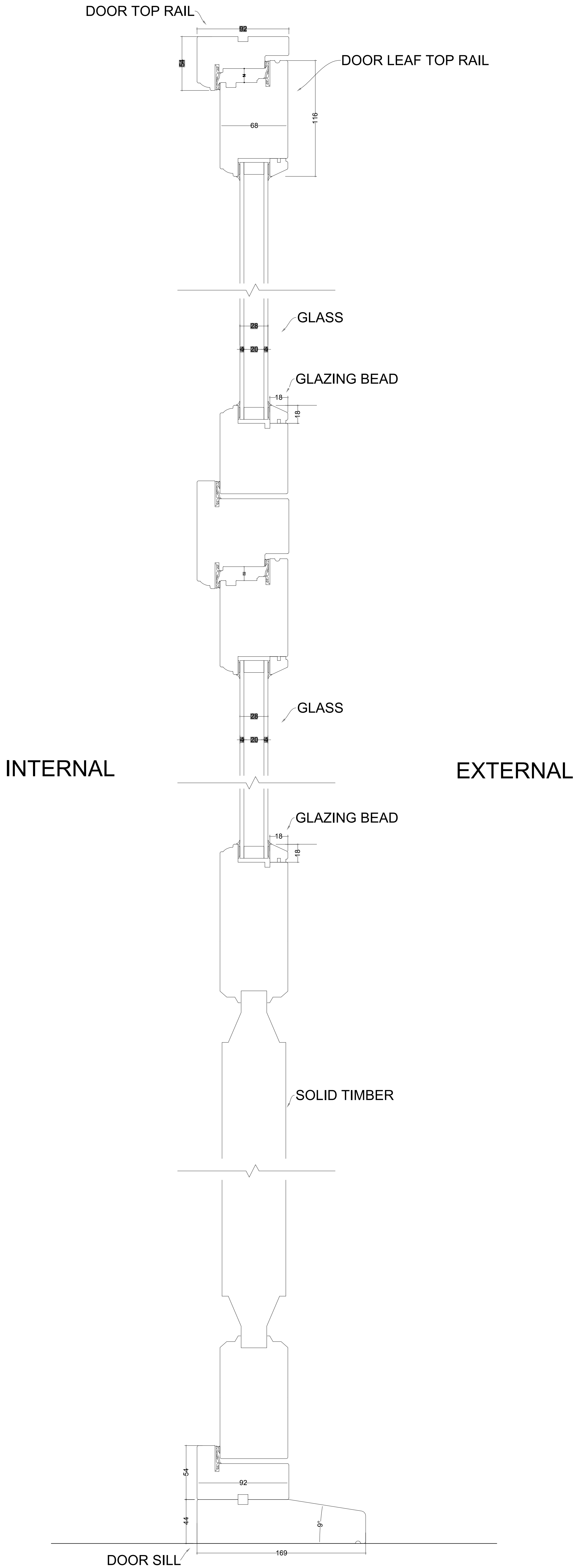
1:2 VERTICAL DOOR SECTION
