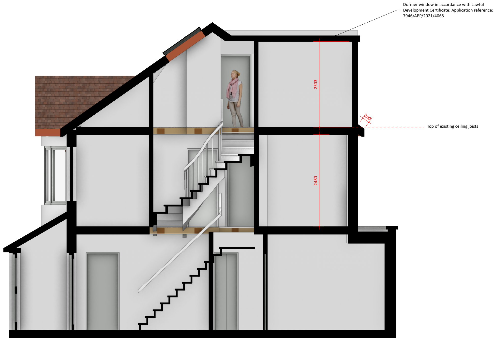
1 SECTION A-A
