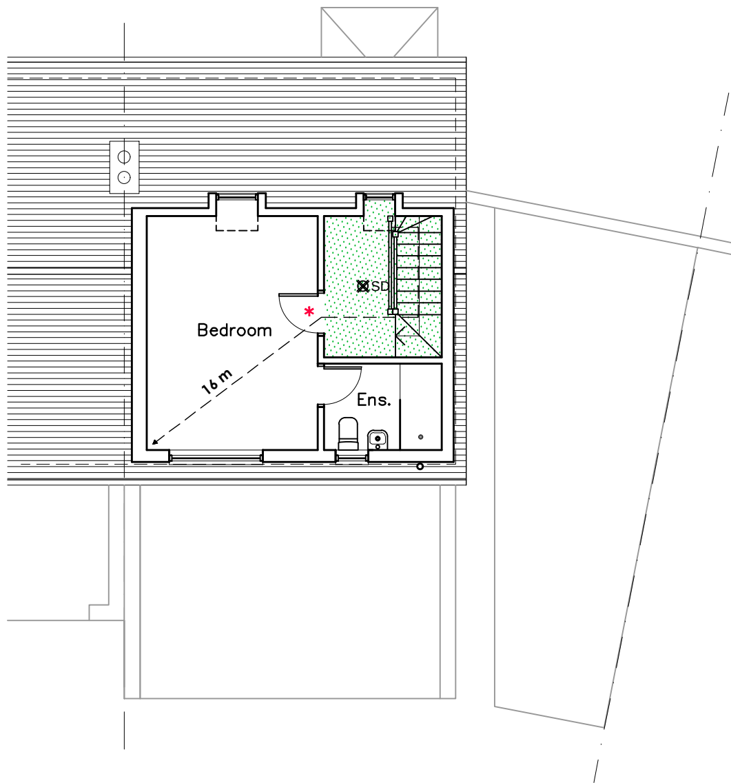
LOFT PLAN
