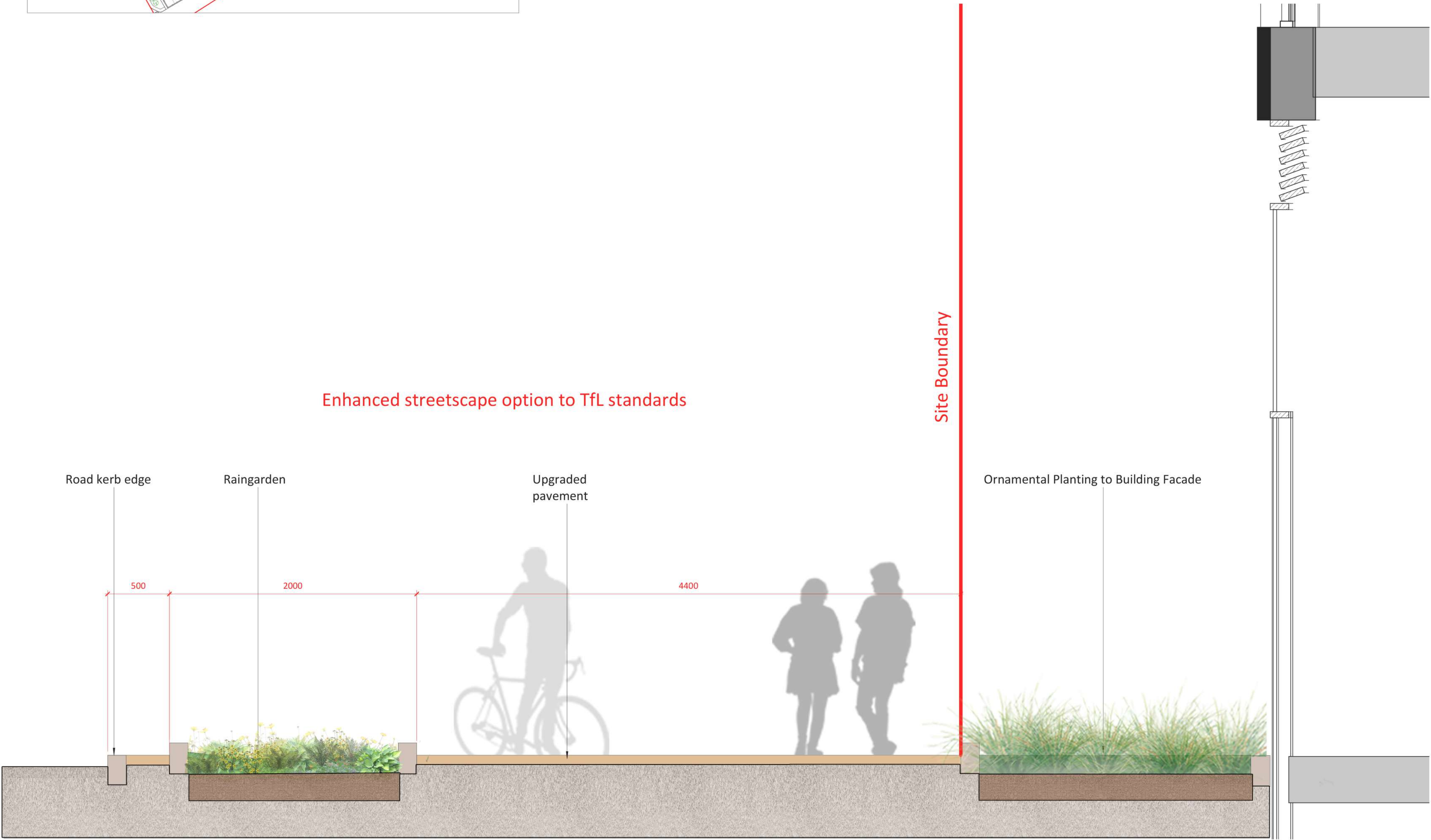
Section 2 - Street 1 : 20
