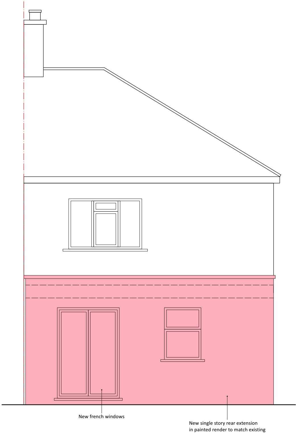
1 South Elevation Scale: 1:50
