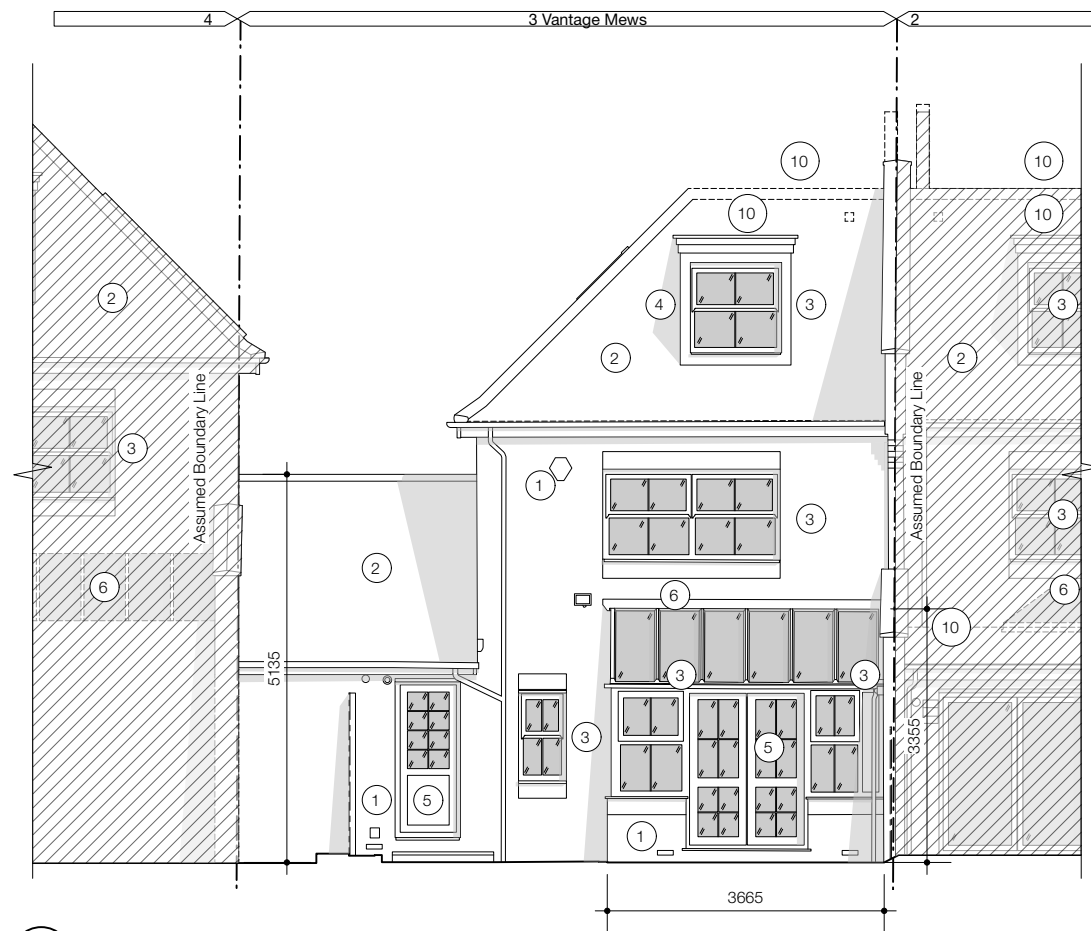
2 Existing Rear Elevation Scale: 1:100
