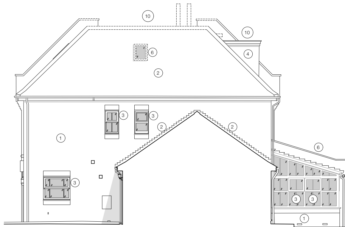
3 Existing Side Elevation Scale: 1:100
