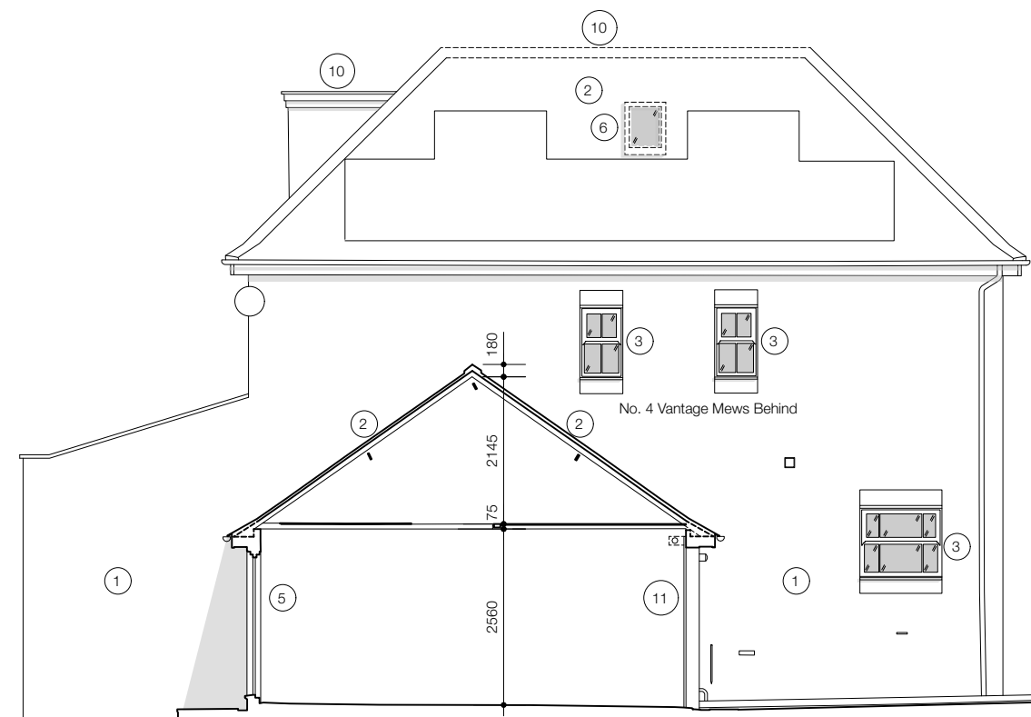
4 Existing Section AA Scale: 1:100
