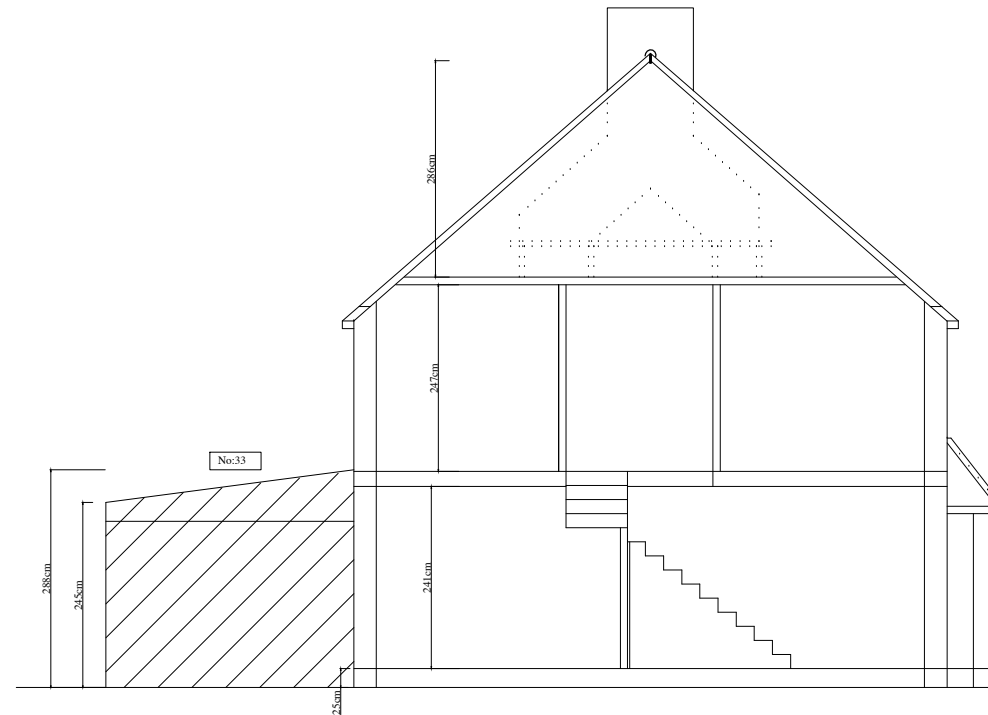
SECTION A-A
