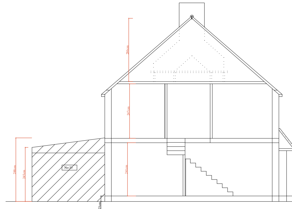
SECTION A-A
