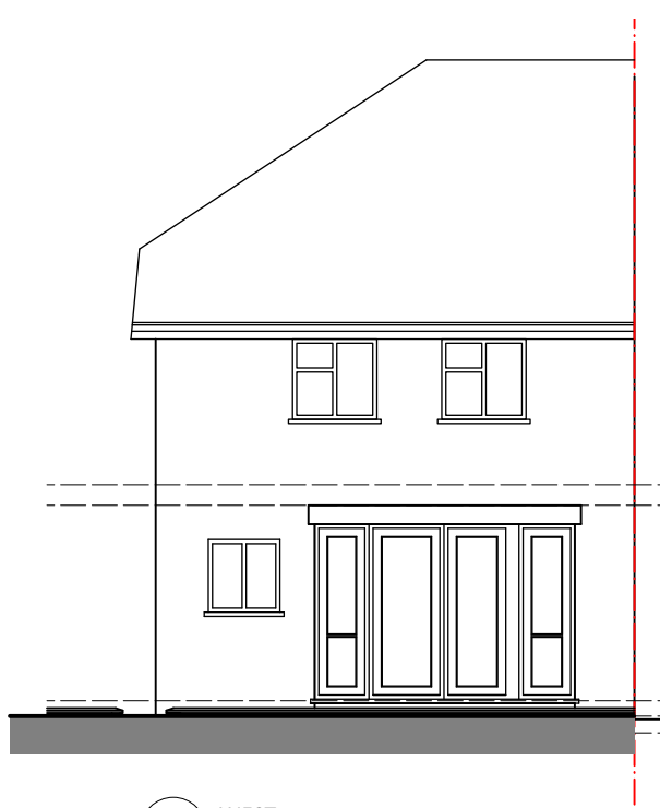
3 WEST Scale: 1:100
