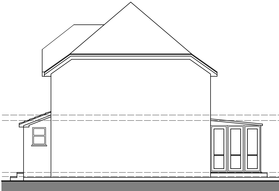
4 NORTH Scale: 1:100
