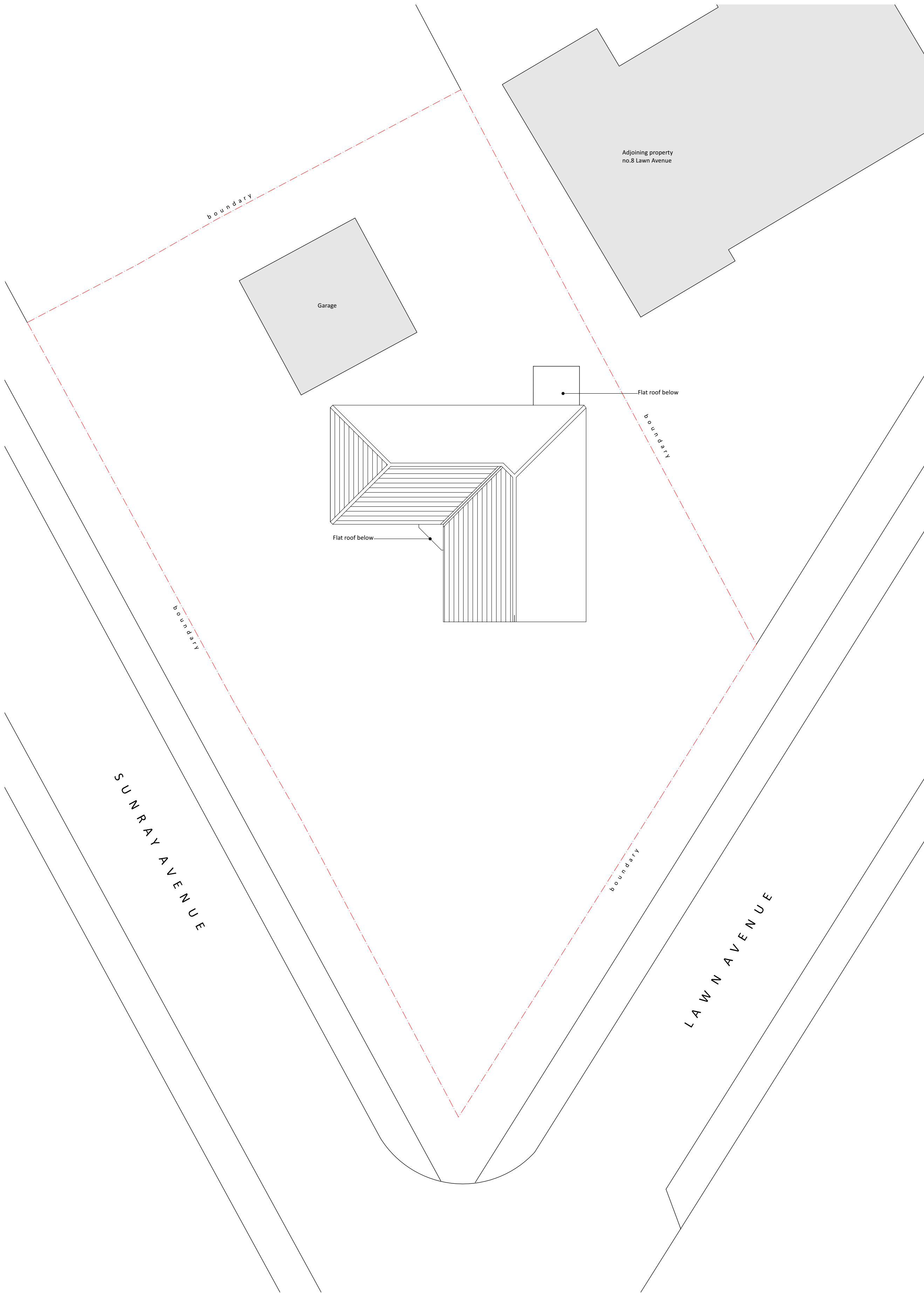
1 ROOF Scale: 1:100
