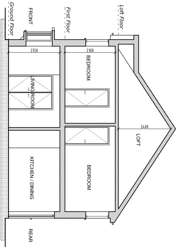
Section A-A
