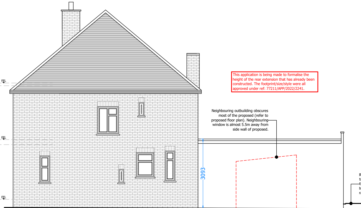
FLANK ELEVATION
