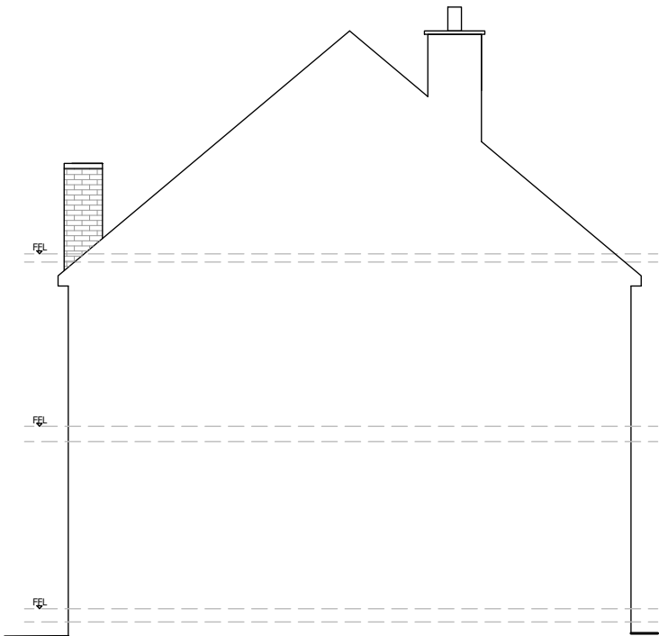
FLANK ELEVATION
