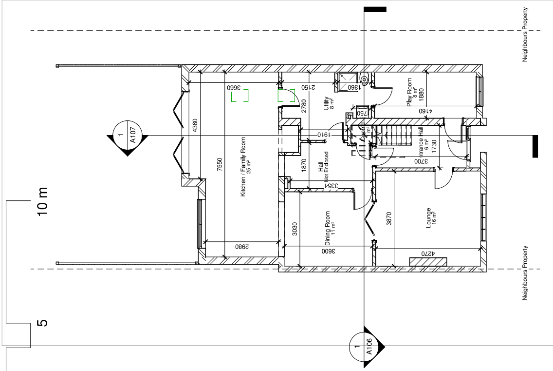
1 00 - Existing 1 : 100
