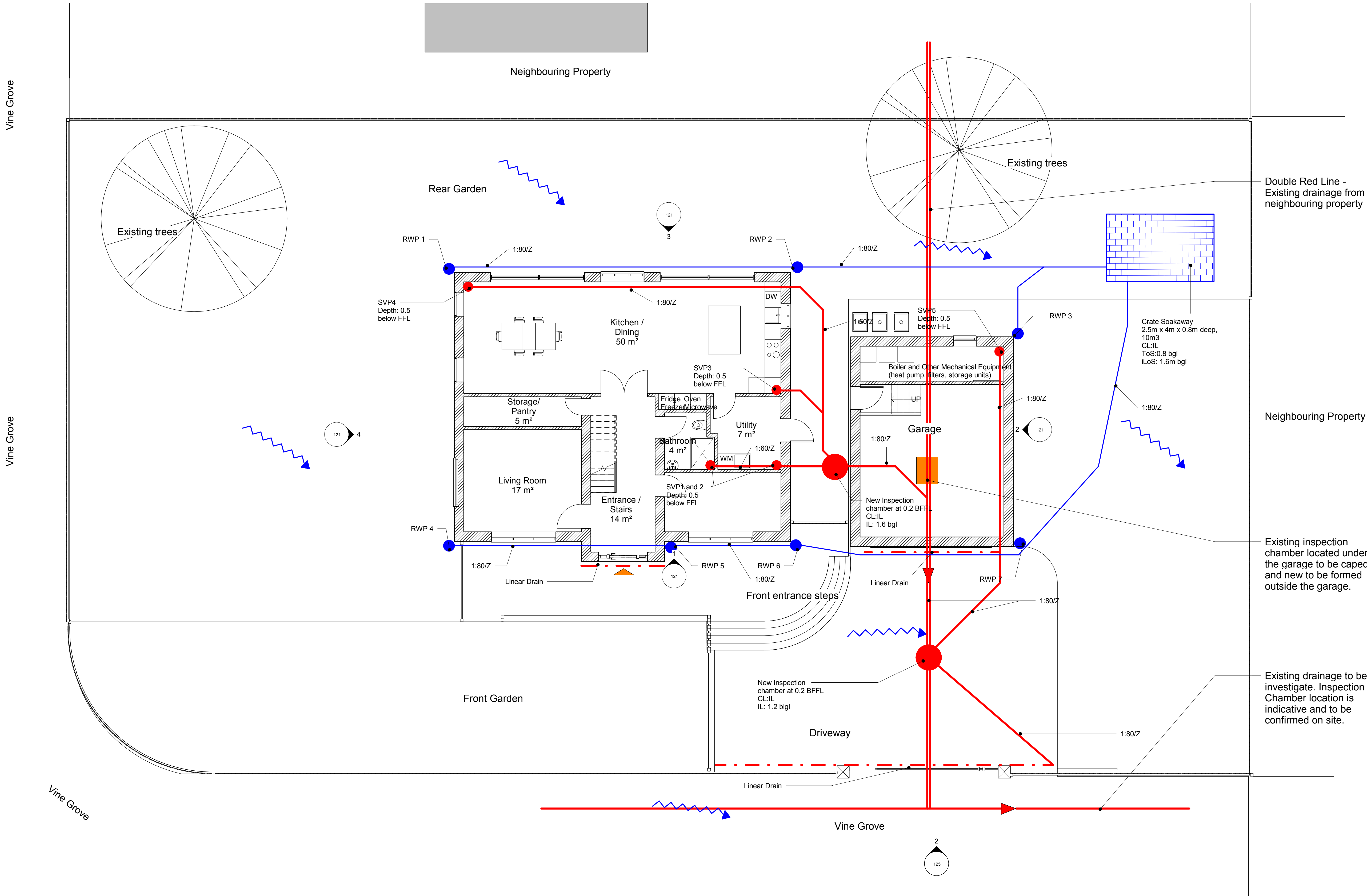
1 DRAINAGE PLAN 1 : 75
