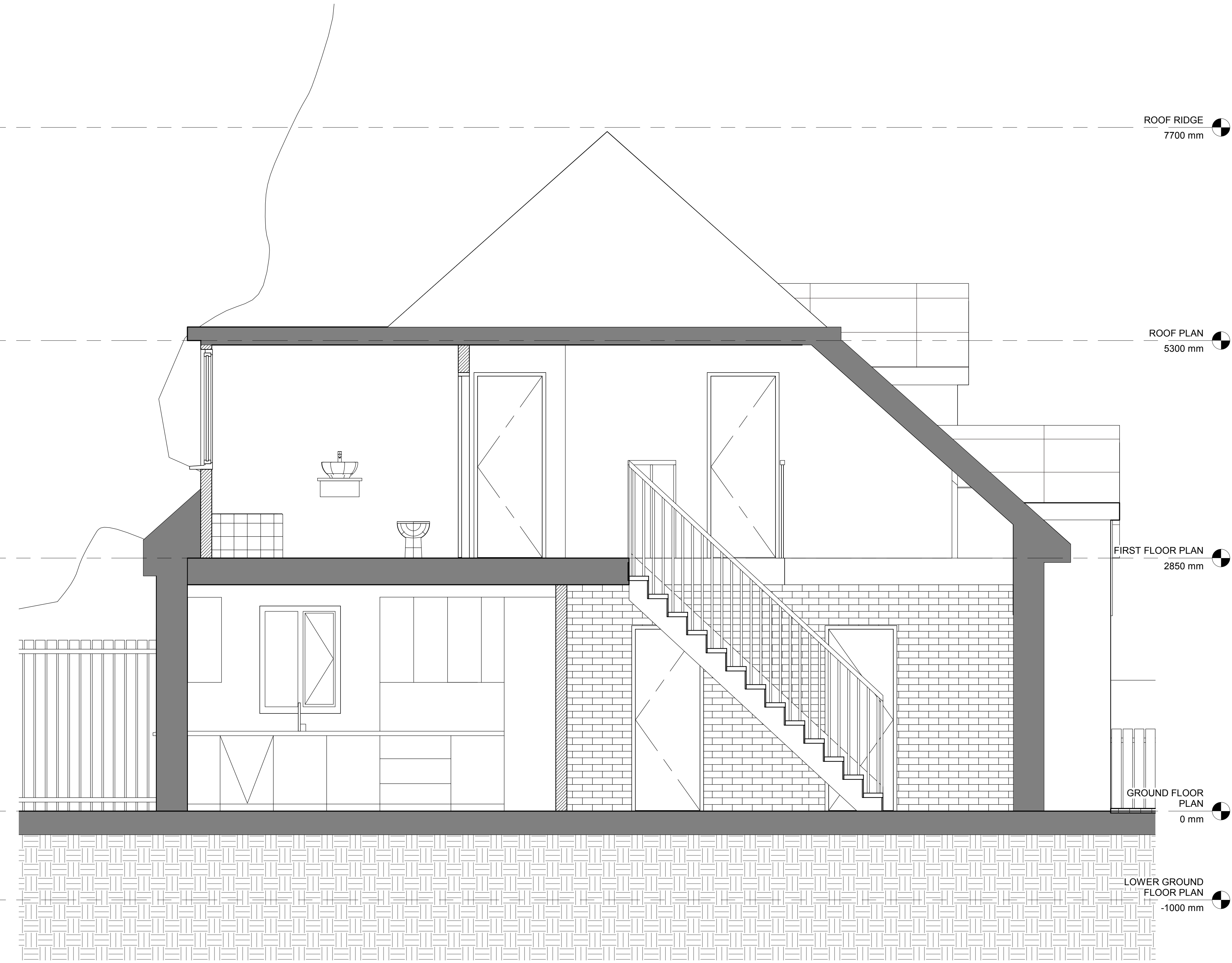
1 Section AA 1 : 25
