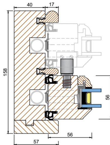
Section A-A - Top Sash Jamb
