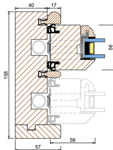
Section C-C - Bottom Sash Jamb
