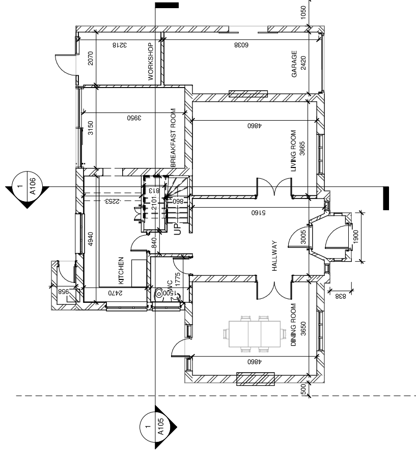
1 00 - Existing 1 : 100
