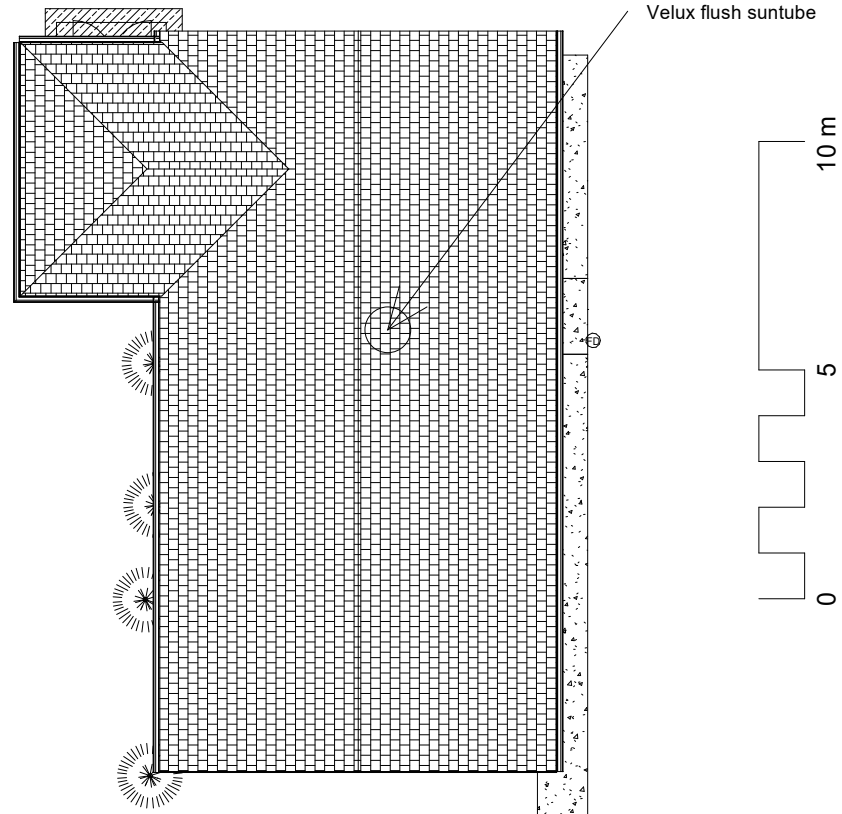
2 Prop Roof 1 : 100
