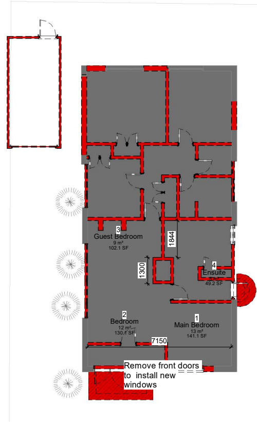
1 Demolition 1 : 100
