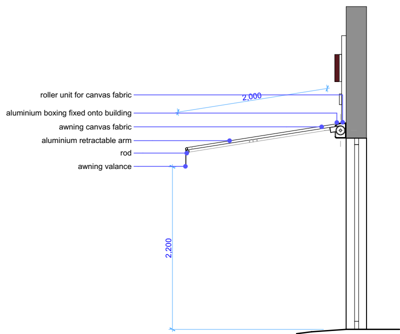
Awning Section 1:50
