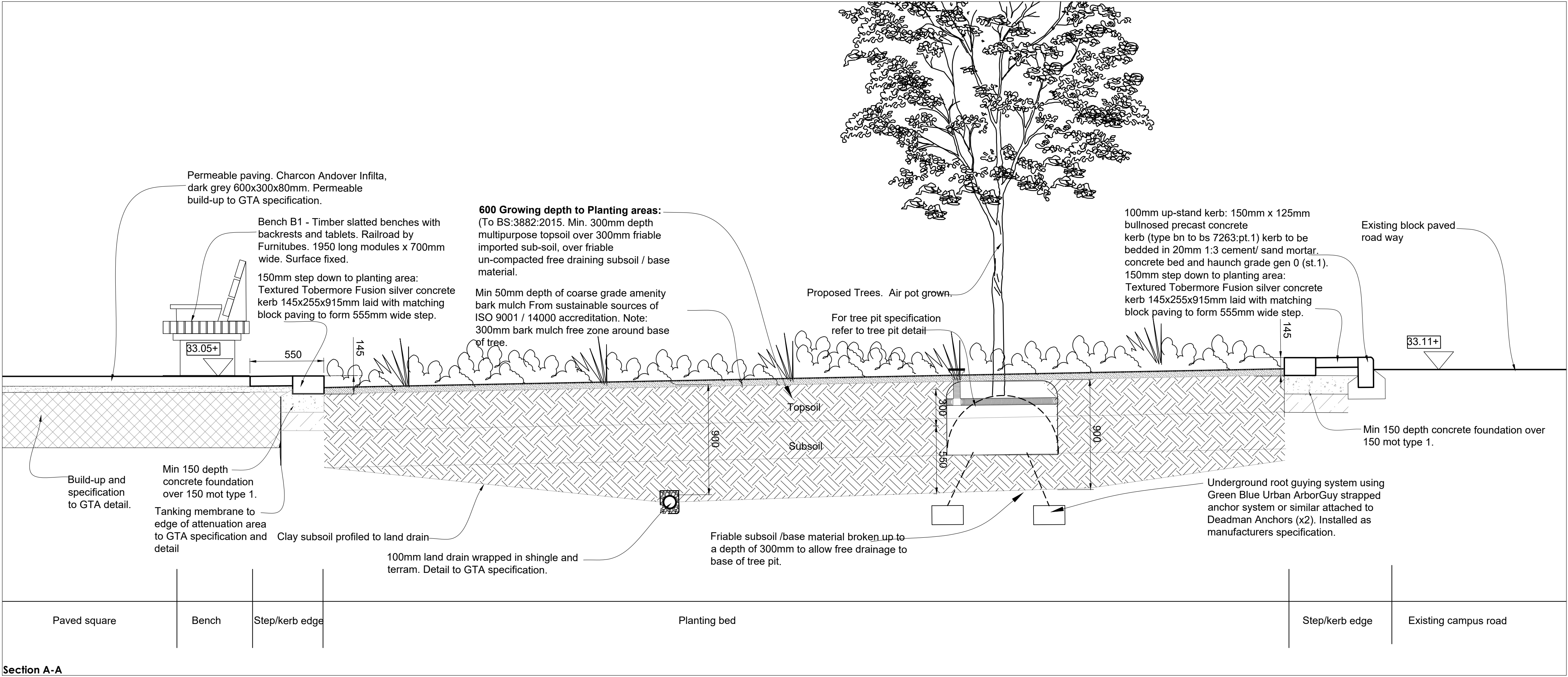
Section A-A Scale 1:20@A1
