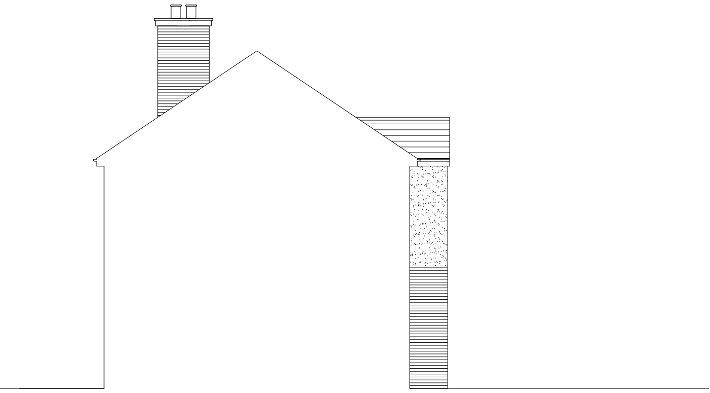
2 SIDE ELEVATION - EXISTING Scale: 1:100
