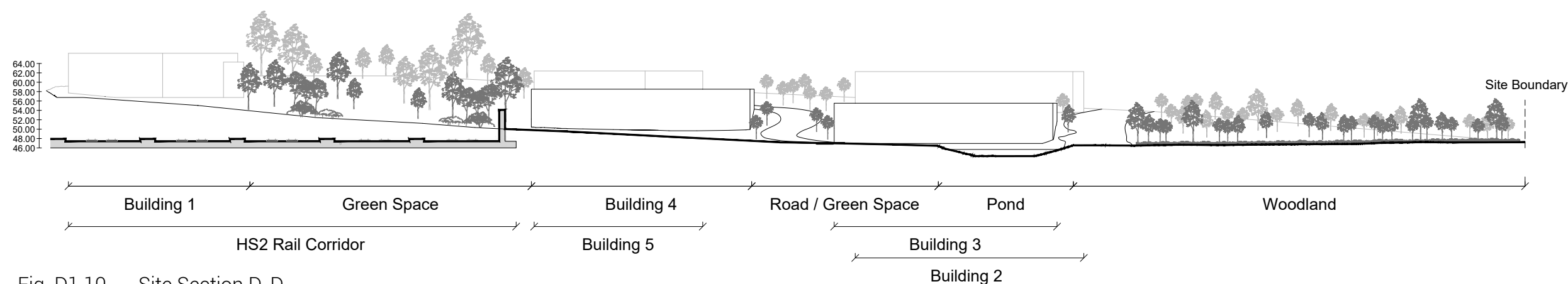
Fig. D1.10 Site Section D-D
