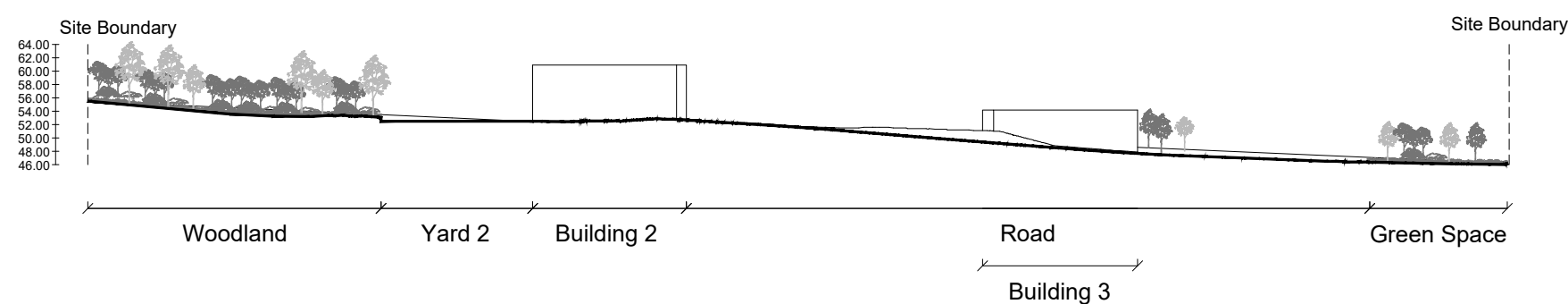
Fig. D1.11 Site Section E-E
