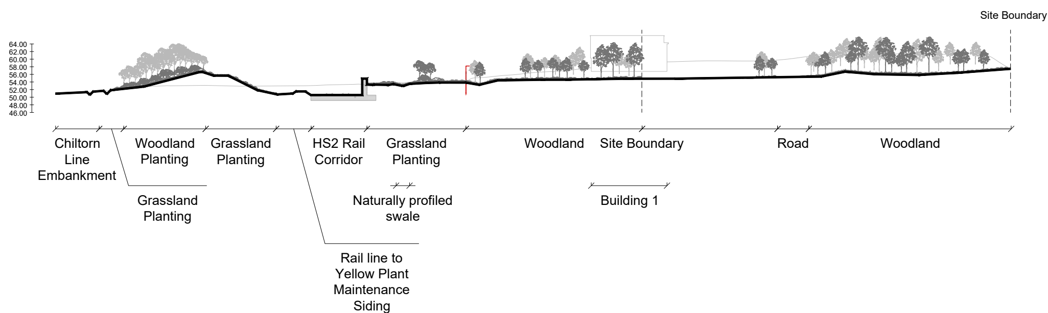
Fig. D1.12 Site Section F-F
