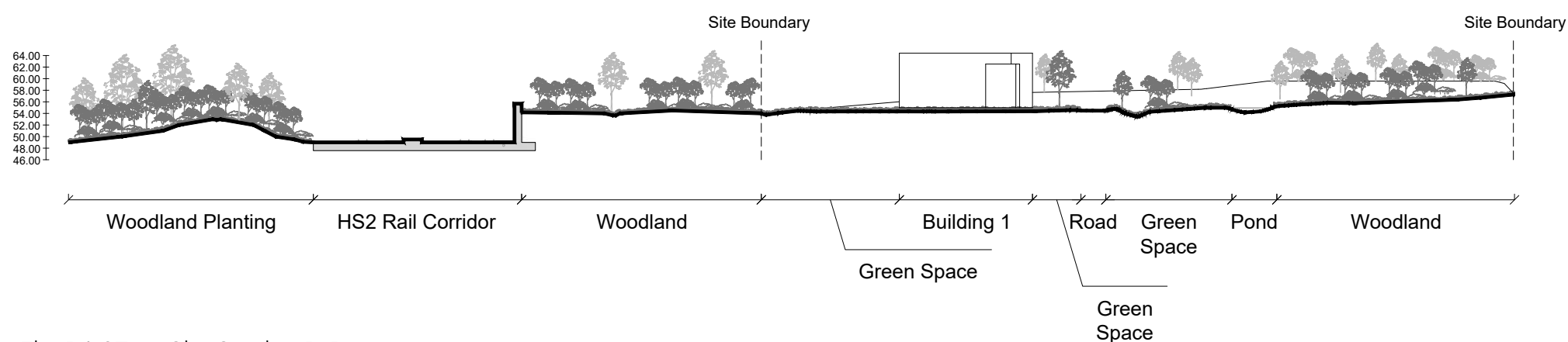
Fig. D1.07 Site Section B-B
