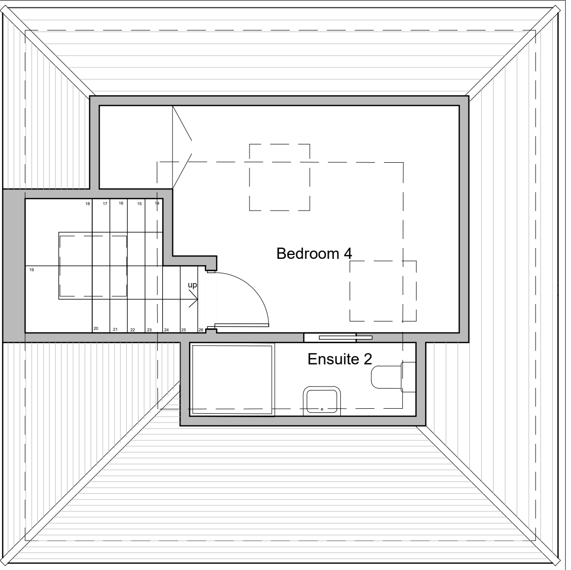
LOFT
