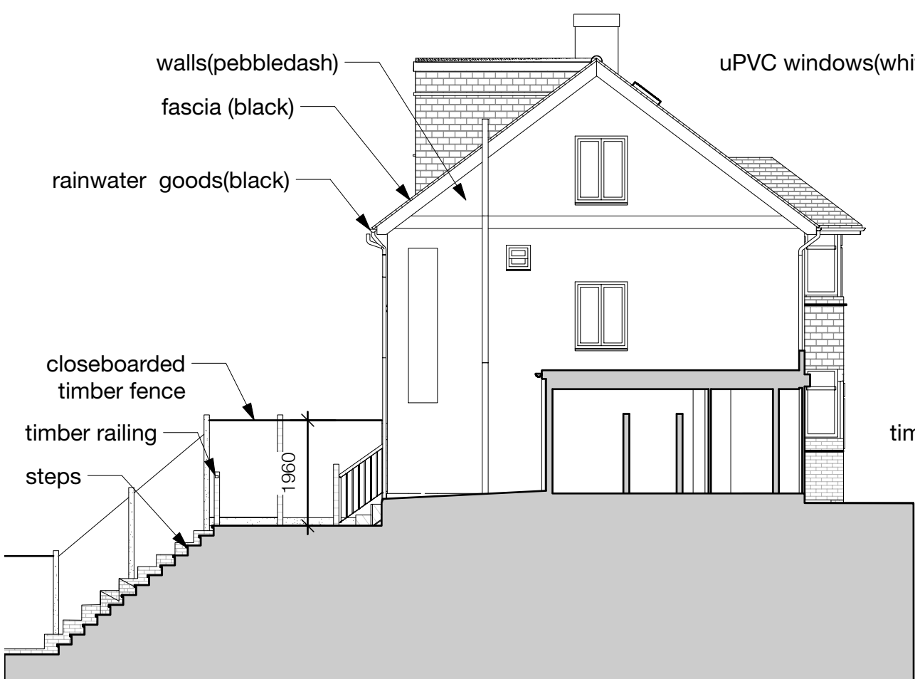
01 Flank Elevation to no 72 Scale: 1:100
