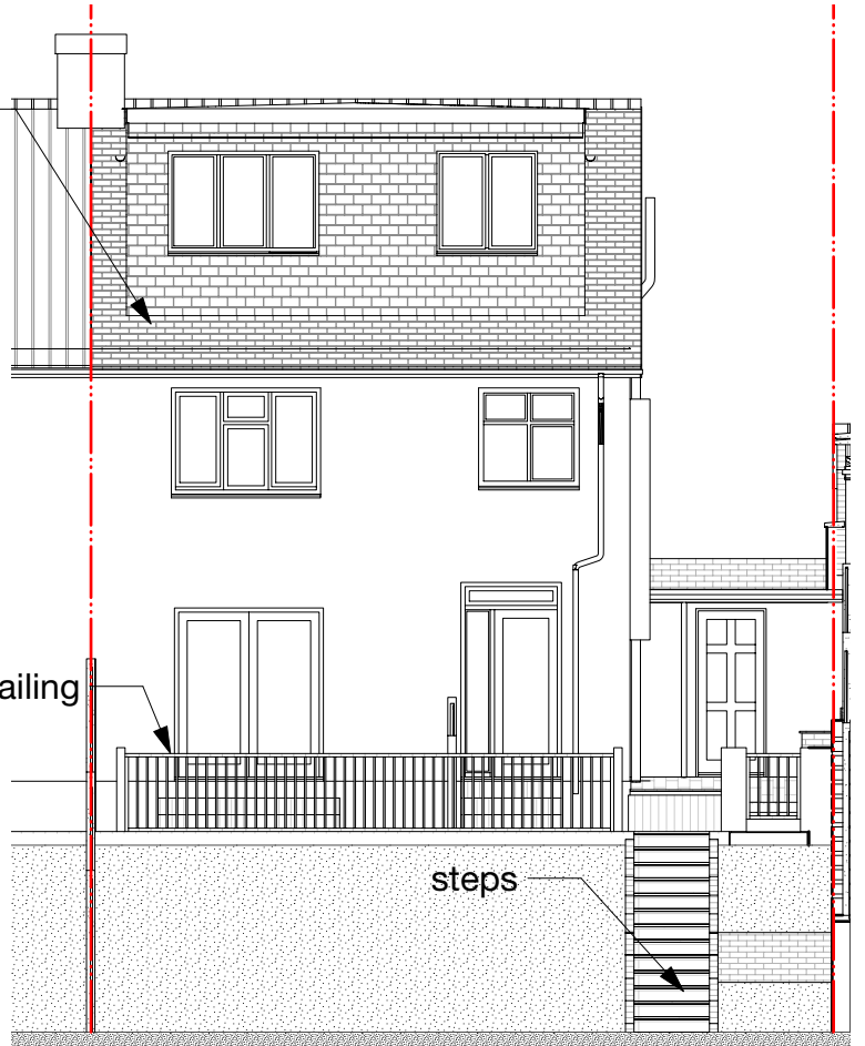
02 Rear Elevation Scale: 1:100
