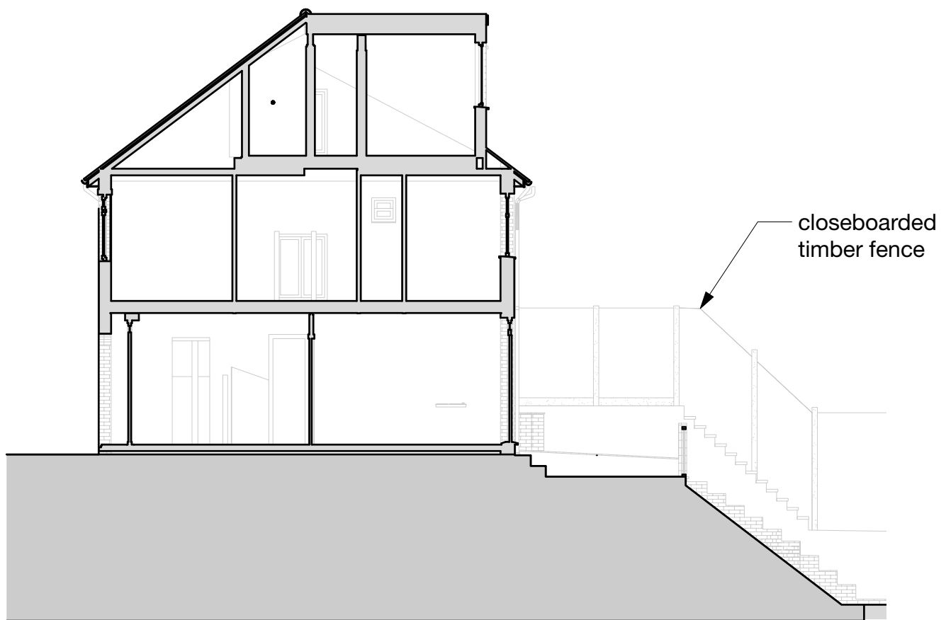
05 Section AA Scale: 1:100
