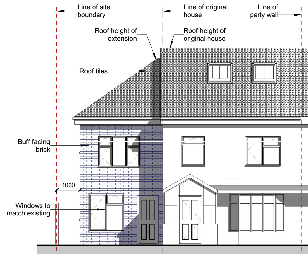
1 Front Elevation Option 2 1910-A-311 1 : 100
