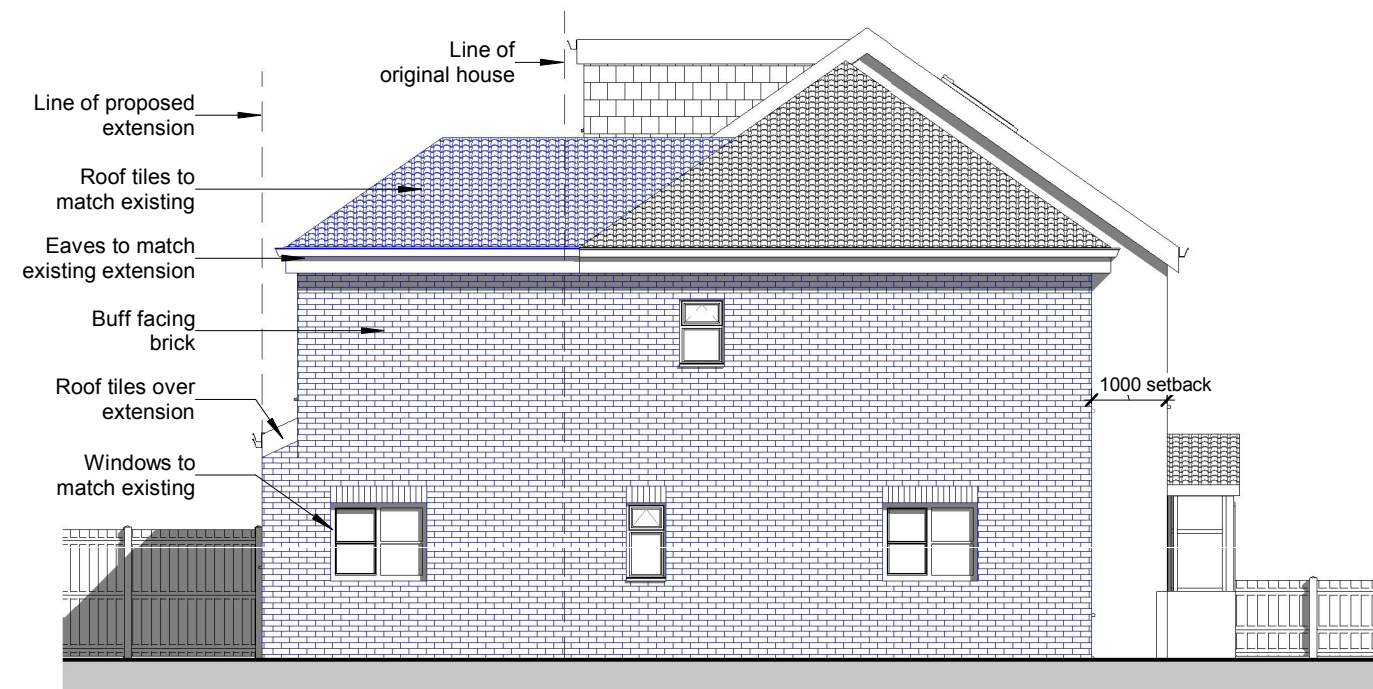
3 Side Elevation Option 2 1910-A-311 1 : 100
