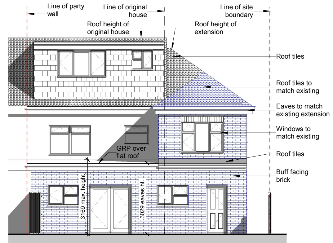
2 Rear Elevation Option 2 1910-A-311 1 : 100
