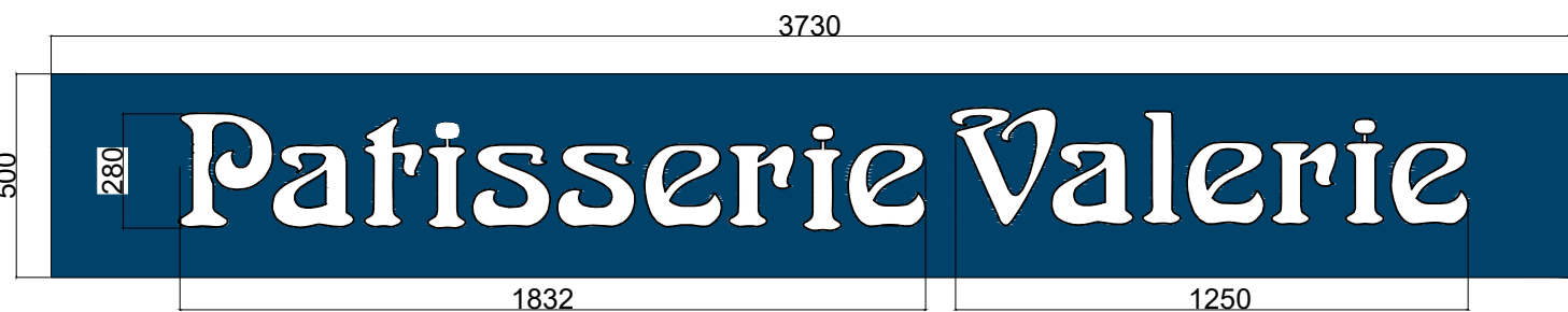
1 EXTERNAL FASCIA SIGN Scale: 1:20
