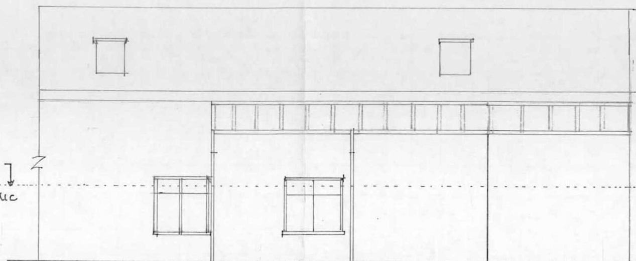
ELEVATION — (B) — 1:100
