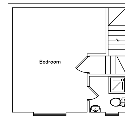
Loft Plan
