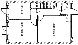
00 - Existing 1 : 100
