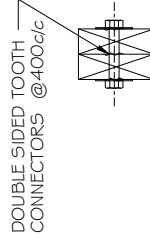
DOUBLE - UP JOISTS(d)
