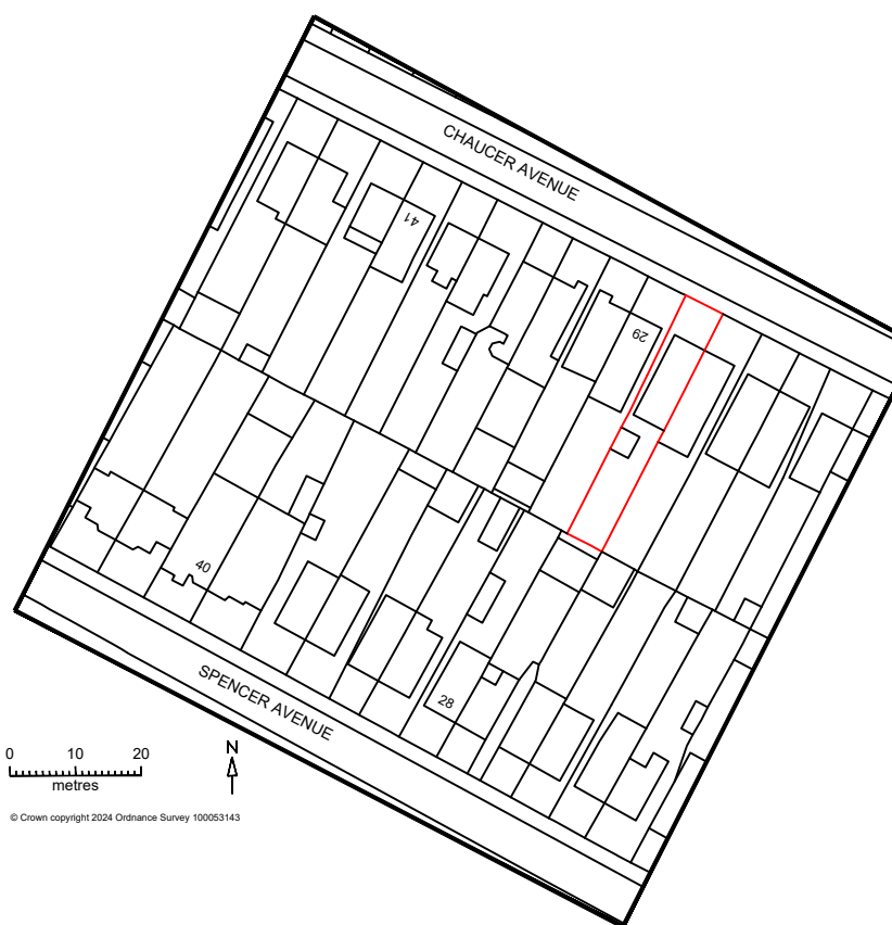
Site Plan 1 : 1250 27 Chaucer Ave, Hayes UB4 0AP
