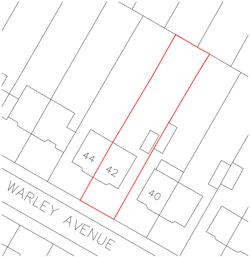
SITE PLAN 1/500
