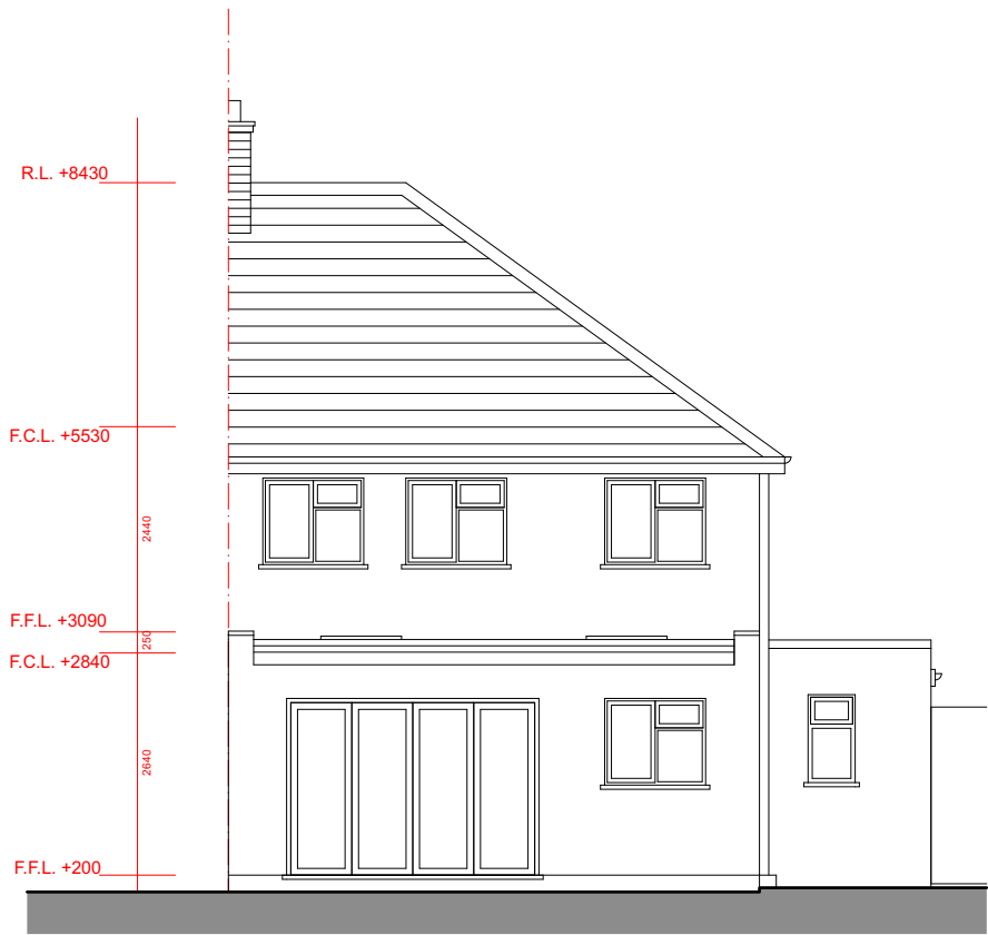
1 WEST - Rear Scale: 1:100
