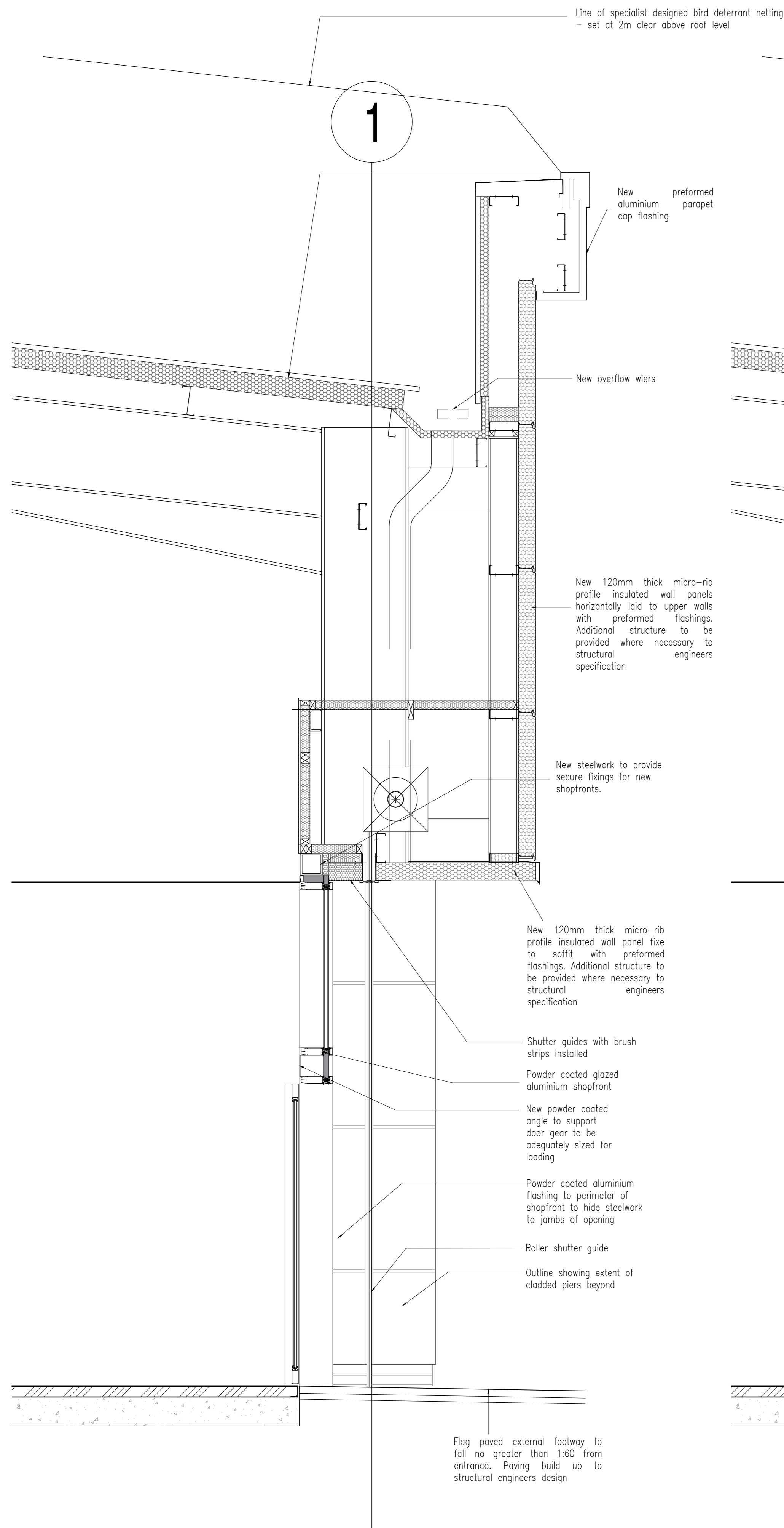
SECTION 1-1 1:20
