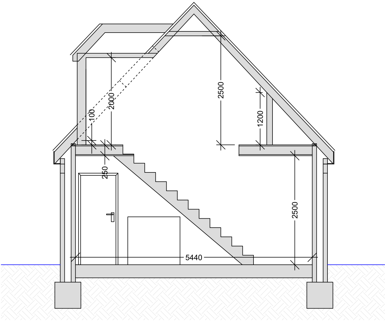
○ Section A - A 1 : 5 0
