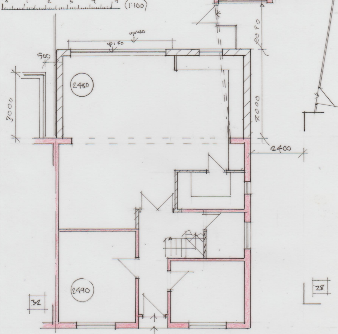
G.F. PLAN 1:100
