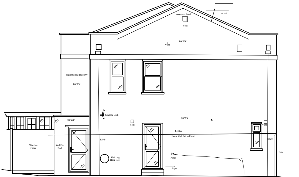
Elevation 4
