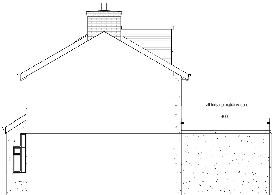
AE-0020-01 - Side Elevation
