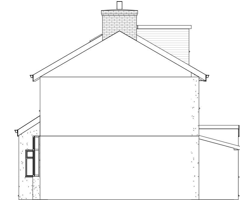
AE-0020-01 - Side Elevation
