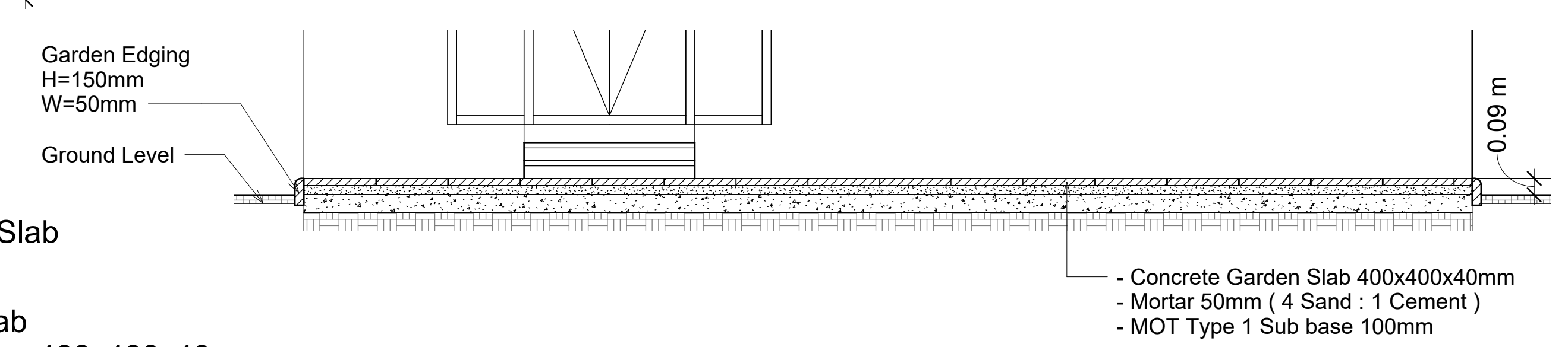
Section A-A Scale 1:25
