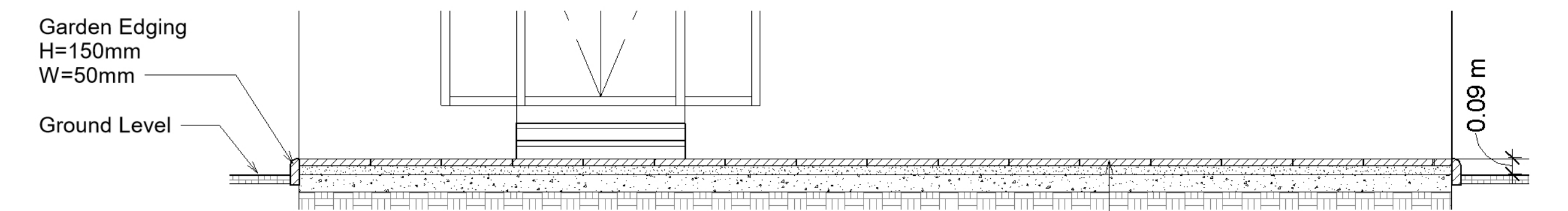
Section A-A Scale 1:25
