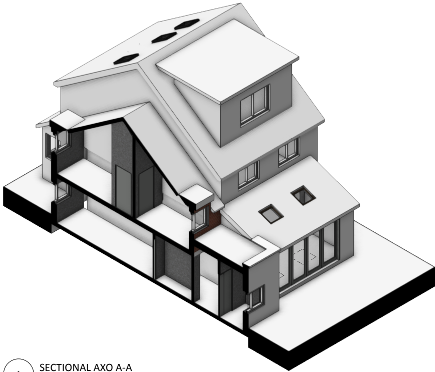
1 SECTIONAL AXO A-A Scale: NTS
