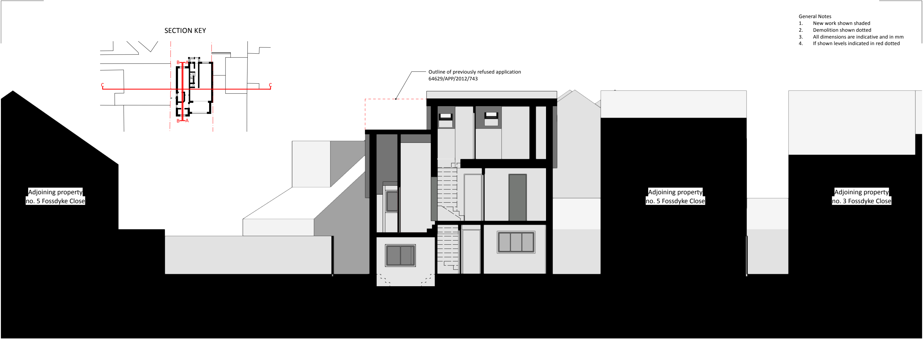
3 SECTIONAL C-C Scale: 1:100
